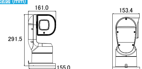
外形寸法図 (mm)
